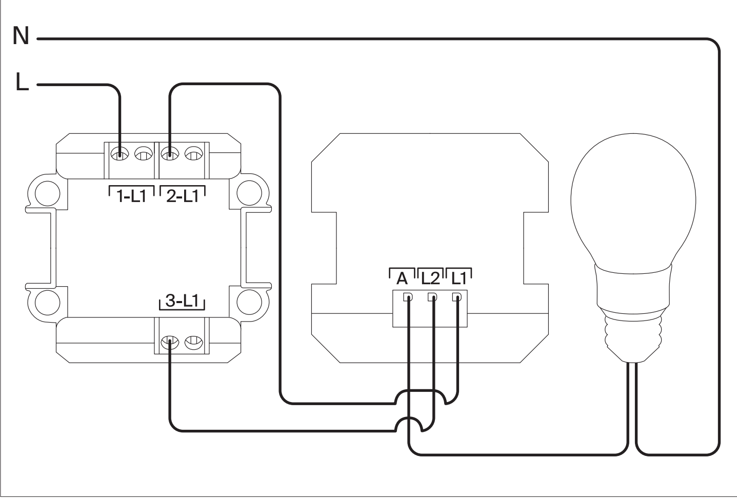
Схема подключения светорегулятора поворотного-нажимного и проходного выключателя одноклавишного
